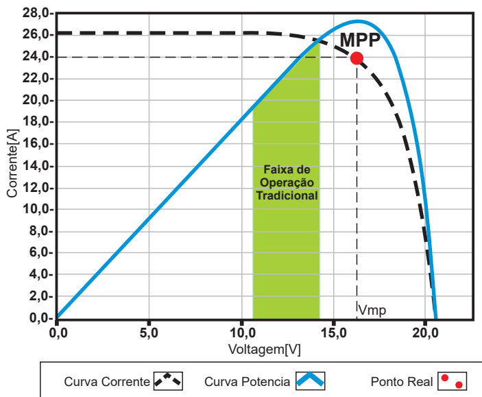
Curva Máximo Ponto de Potencia
